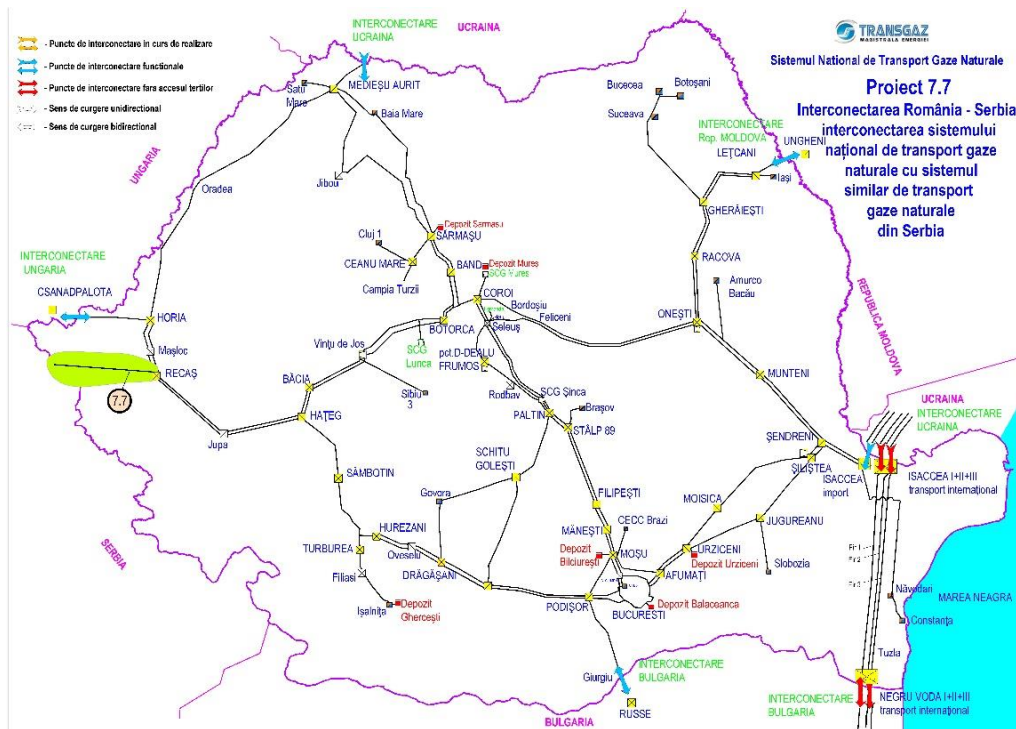
Figura 14 - Interconectarea SNT cu Serbia pe direcția Recea–Mokrin
